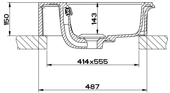
SEZIONE B-B
