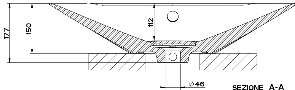
LAVABO D'APPOGGIO COUNTER WASHBASIN
